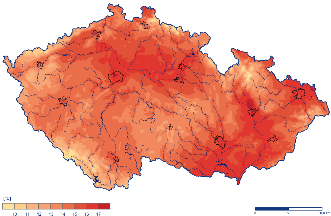
Obr. 2.1.1 Průměrná měsíční teplota vzduchu na území ČR v květnu 2024
