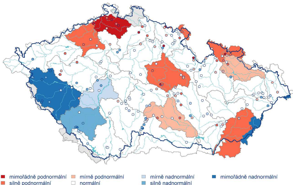
Obr. 3.2.4 Stav vydatnosti pramenů v červnu 2024 a ve skupinách povodí III. řádu. Vztaheno k referenčnímu období 1991–2020.
