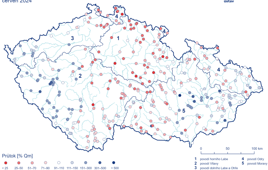
Obr. 3.1.1 Průměrné měsíční průtoky na území ČR, červen 2024
