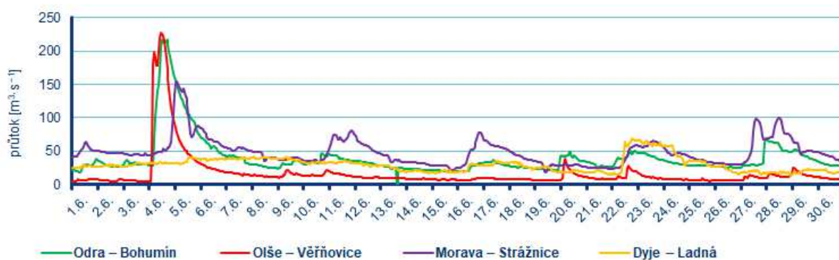
Obr. 3.1.3 Průběh průtoků v červnu v závěrových profilech Odry, Olše, Moravy a Dyje
