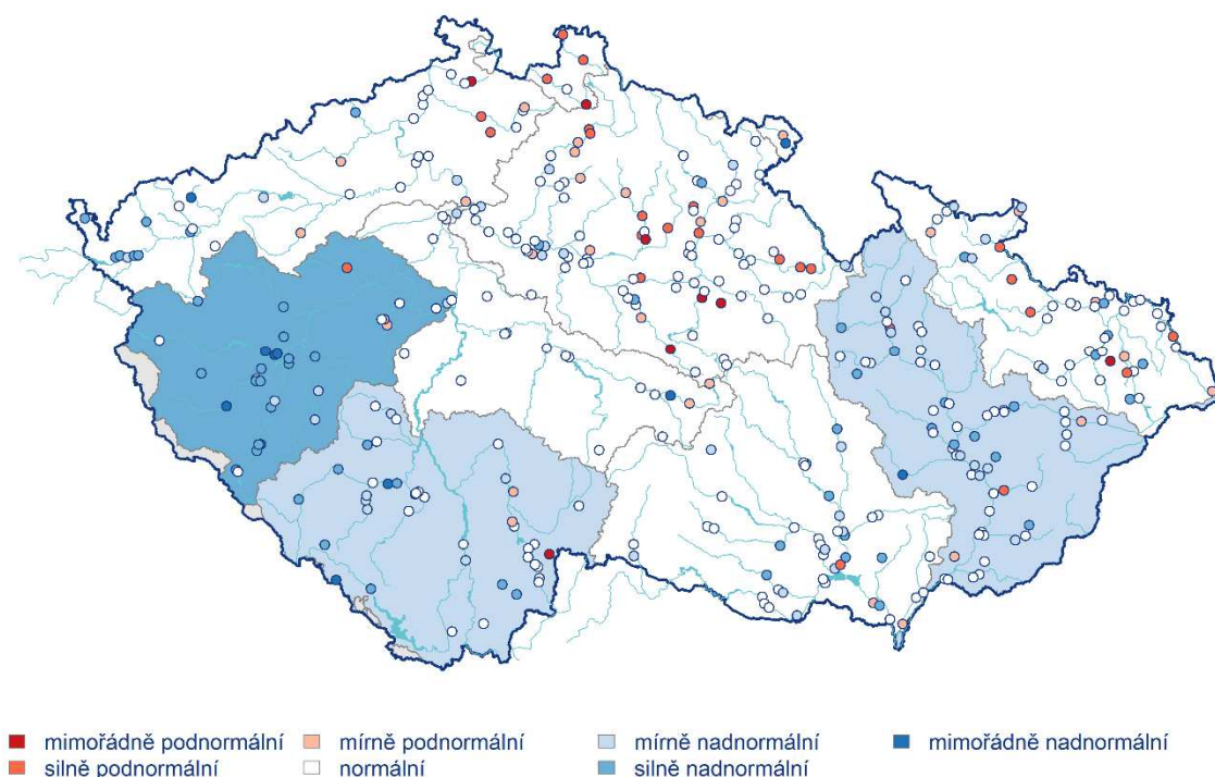
Obr. 3.2.1 Stav hladiny podzemní vody v mělkých vrtech v červnu 2024 v dílčích povodích. Vztaženo k referenčnímu období 1991–2020
