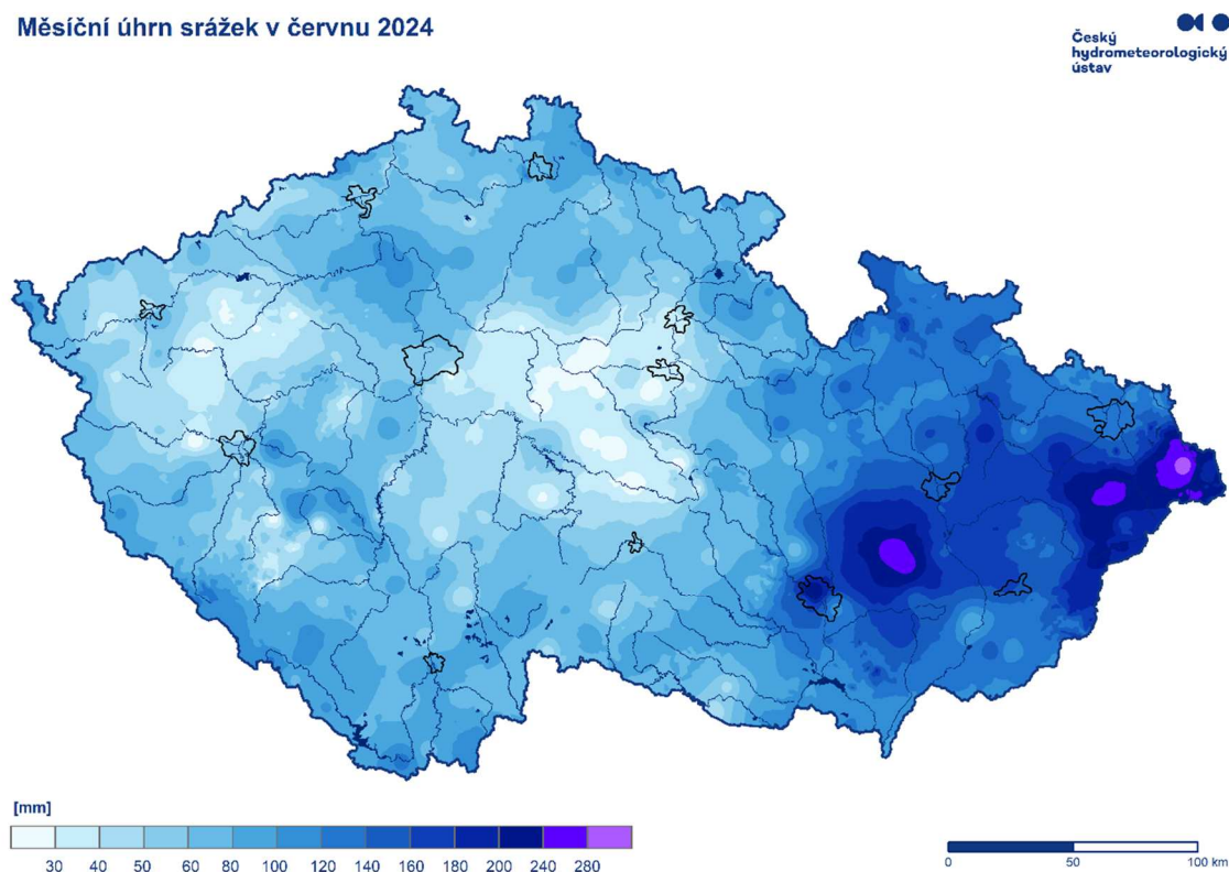
Obr. 2.2.1 Měsíční úhrn srážek na území ČR v červnu 2024
