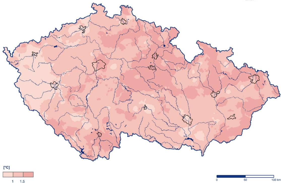
Obr. 2.1.2 Odchylka průměrné měsíční teploty vzduchu od normálu 1991–2020 na území ČR v červnu 2024
