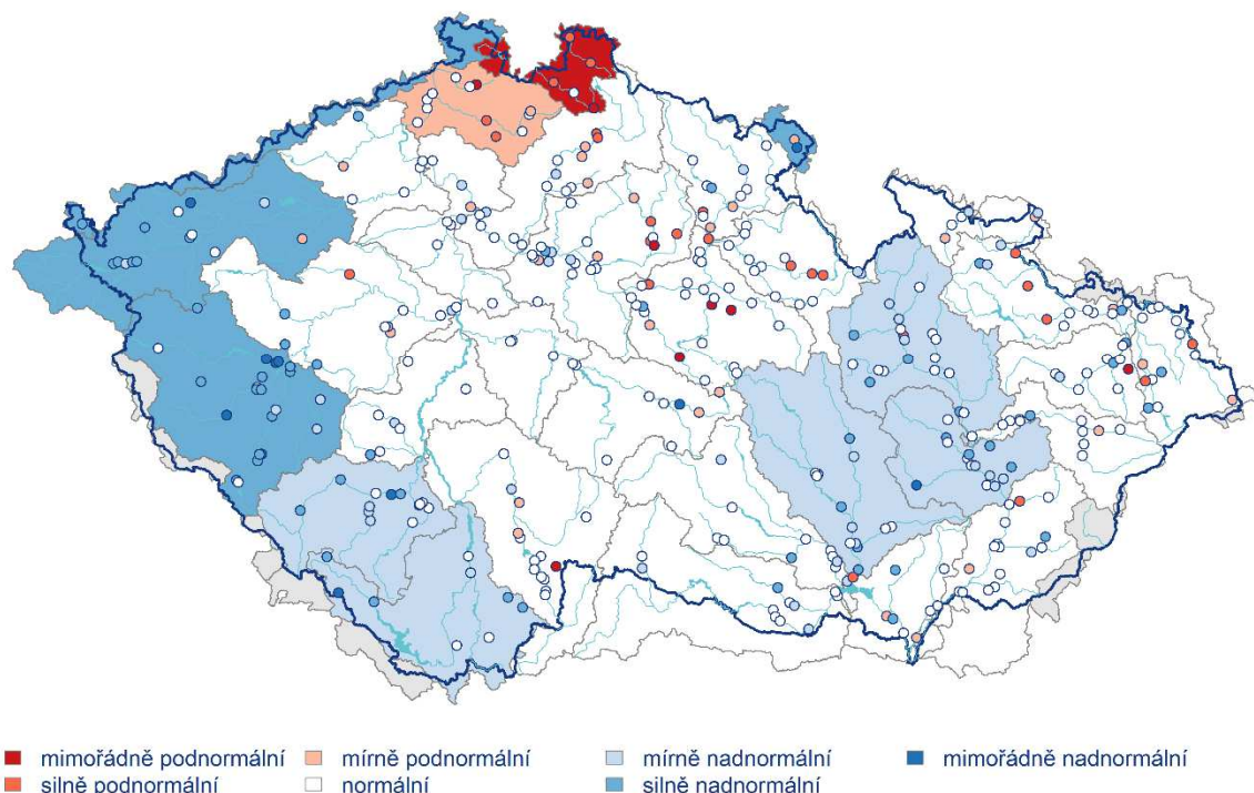
Obr. 3.2.2 Stav hladiny podzemní vody v mělkých vrtech v červnu 2024 a ve skupinách povodí III. řádu. Vztaheno k referenčnímu období 1991–2020
