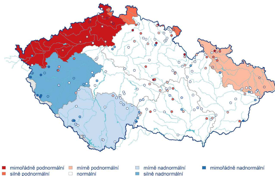
Obr. 3.2.3 Stav vydatnosti pramenů v červnu 2024 v dílčích povodích. Vztaheno k referenčnímu období 1991–2020
