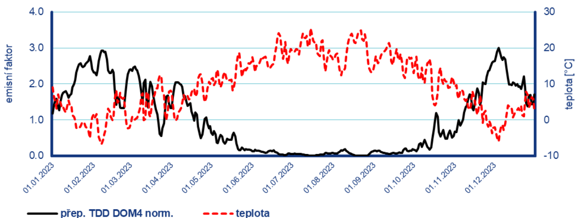
Obr. 27 Rozpočet emise z lokálního vytápění na dny dle přepočtených typových diagramů dodávek plynu (emisním faktorem je násobena průměrná denní emise) a denní průměry teploty z modelu ALADIN, 2023
